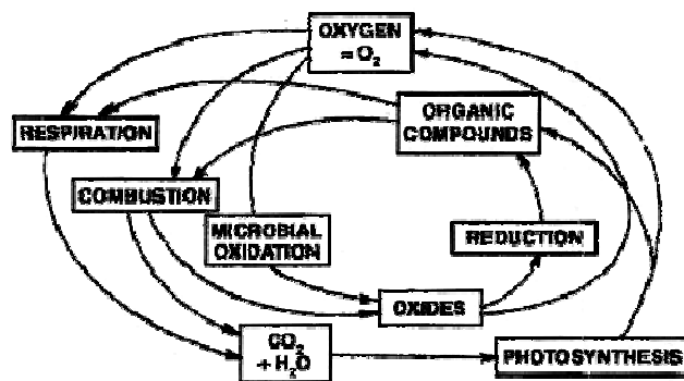
Fig. : Oxygen cycle
