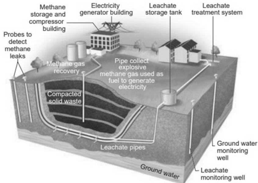
Fig: Sanitary landfill
