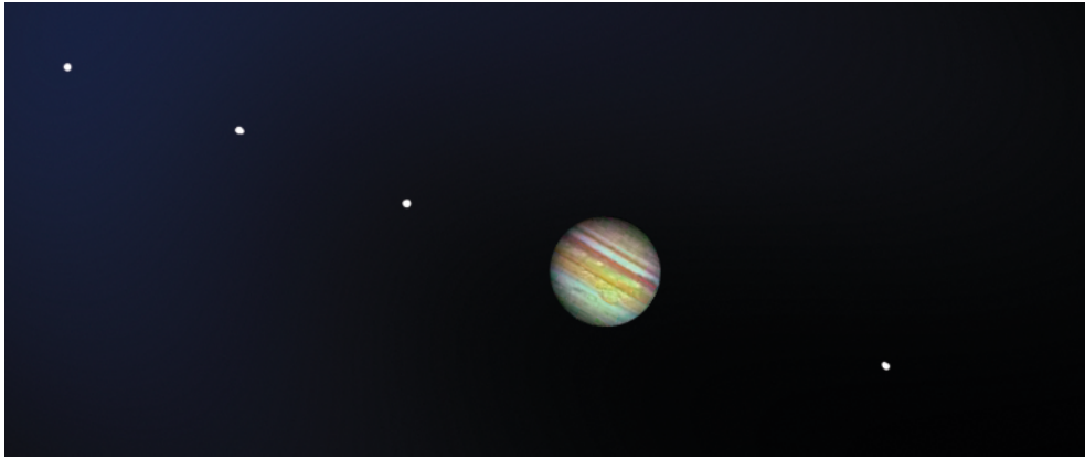
चित्र 17.22 : बृहस्पति और उसके चार बड़े उपग्रह।
