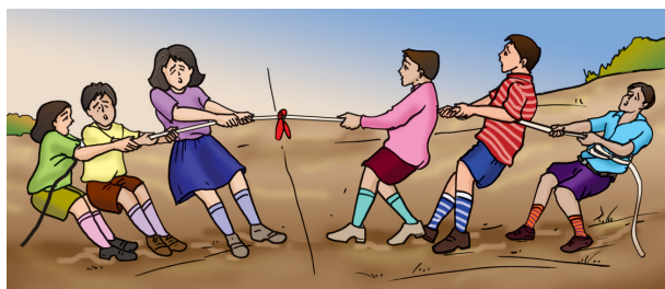
चित्र 11.5 : यदि दोनों टोलियाँ रस्से को समान बल से खींचती हैं तो रस्सा खिसकता नहीं।
