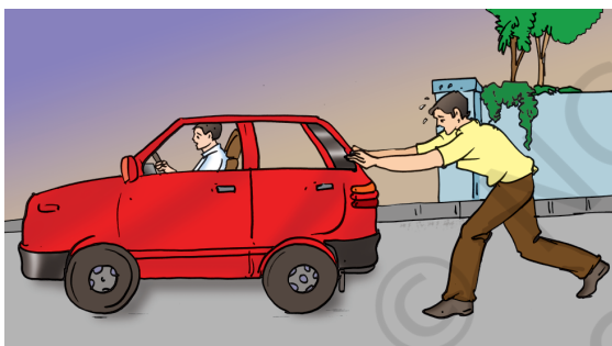
चित्र 11.2(b) : एक आदमी द्वारा कार को धक्का लगाना।
